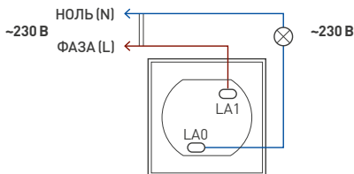
Рис. 1. Схема подключения
