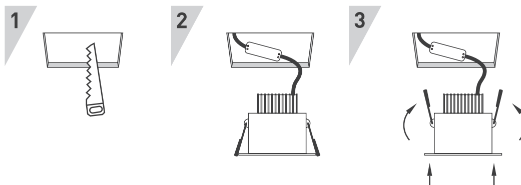
Рис. 2. Установка и подключение светильника
