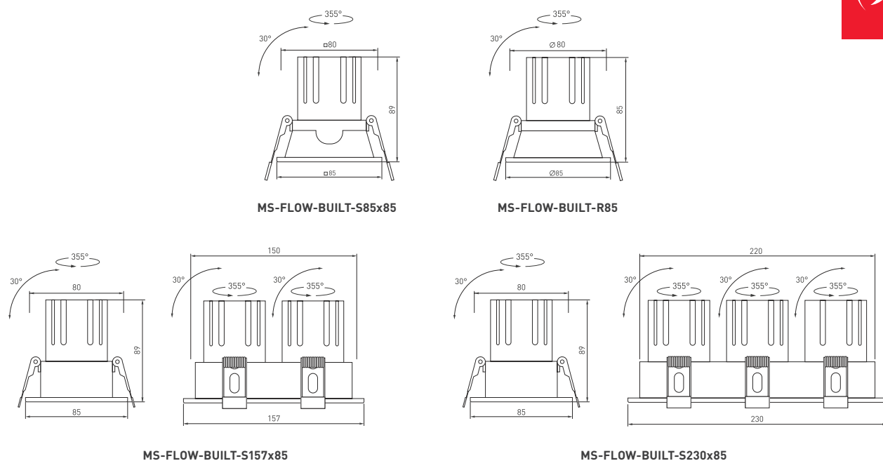
Рис. 1. Чертеж и габаритные размеры
