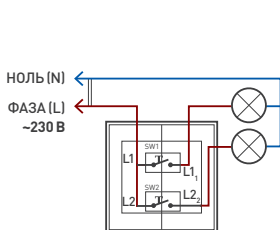
Рис. 1. Схема подключения (арт. 043724, 043725, 043726)
