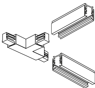
Коннектор T-образный. Внутренняя сторона Арт. 026141/026149
