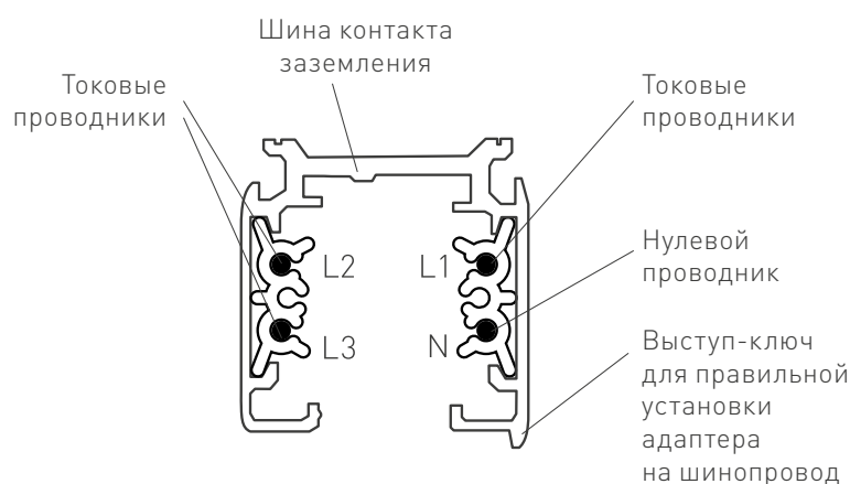
Рис. 1. Конструкция шинопровода
