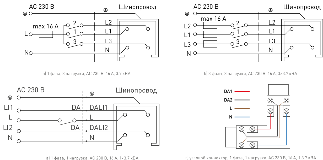
Рис. 3. Схема подключения
