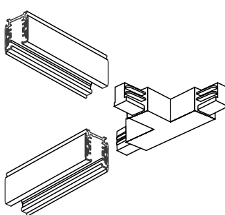
Коннектор T-образный. Внутренняя сторона Арт. 026150/026144
