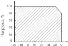
Рис. 3. Максимальная допустимая нагрузка, % от мощности источника
