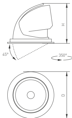
Рис. 1. Чертеж и габаритные размеры
